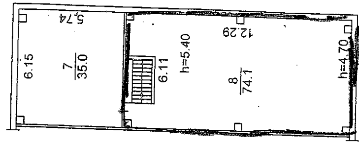
План на отм. 3.000
